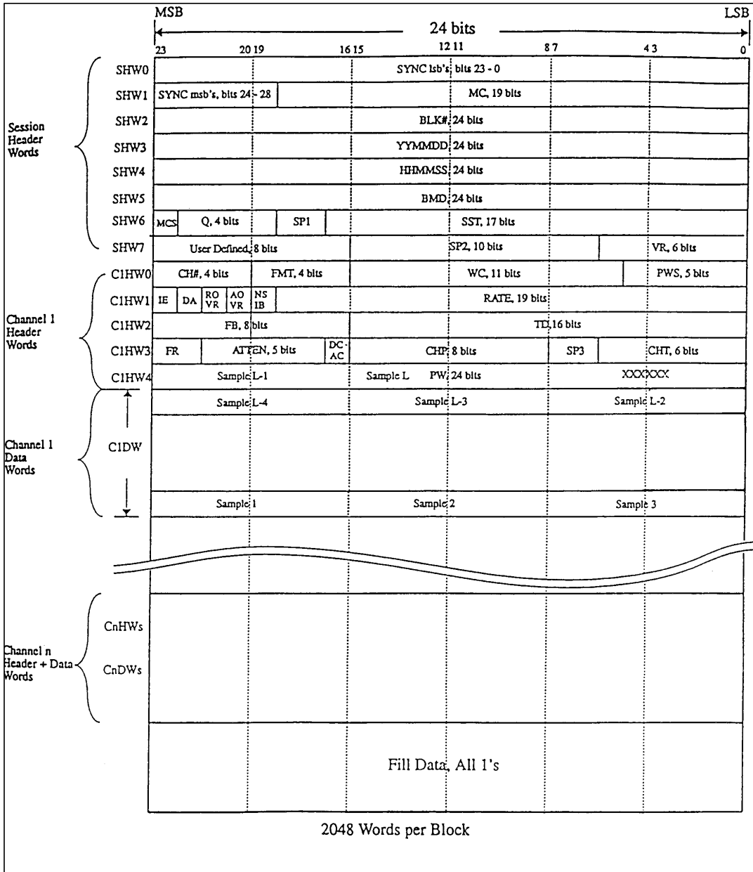
Figure 6-8. ADARIO data format.
