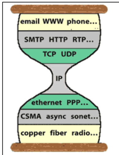
Figure 21-2. IETF Hourglass
