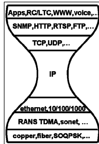
Figure 21-3. TmNS-Specific IETF Hourglass
